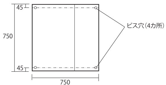
SL-750 固定ビス位置 -W750mm
