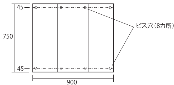
SL-900 固定ビス位置 -W900mm
