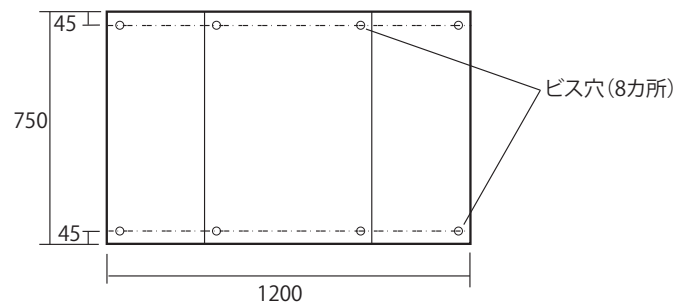
SL-1200 固定ビス位置 -W1200mm
