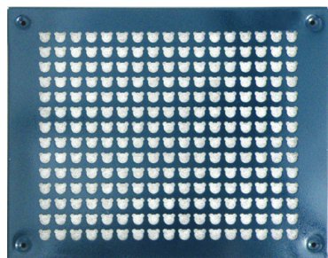
▲ 107F-A2015 サイズ(外寸): W250 H200 D10 カラー(例): 塗装付(指定色)IMビリヤードグリーン
