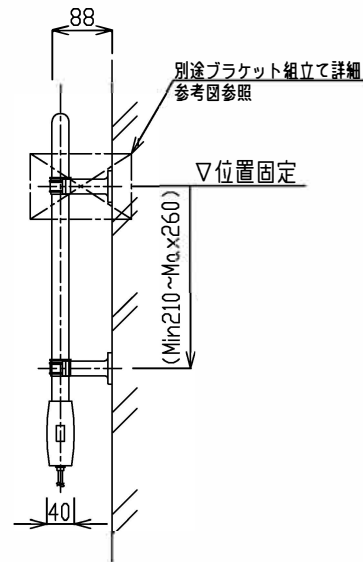
側面(共通)
