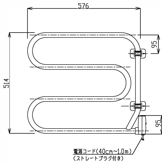
正面(共通)
