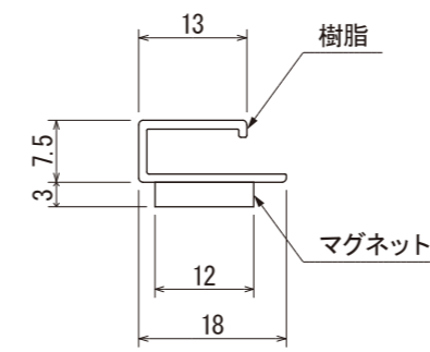
断面詳細図 (S=1/1)
