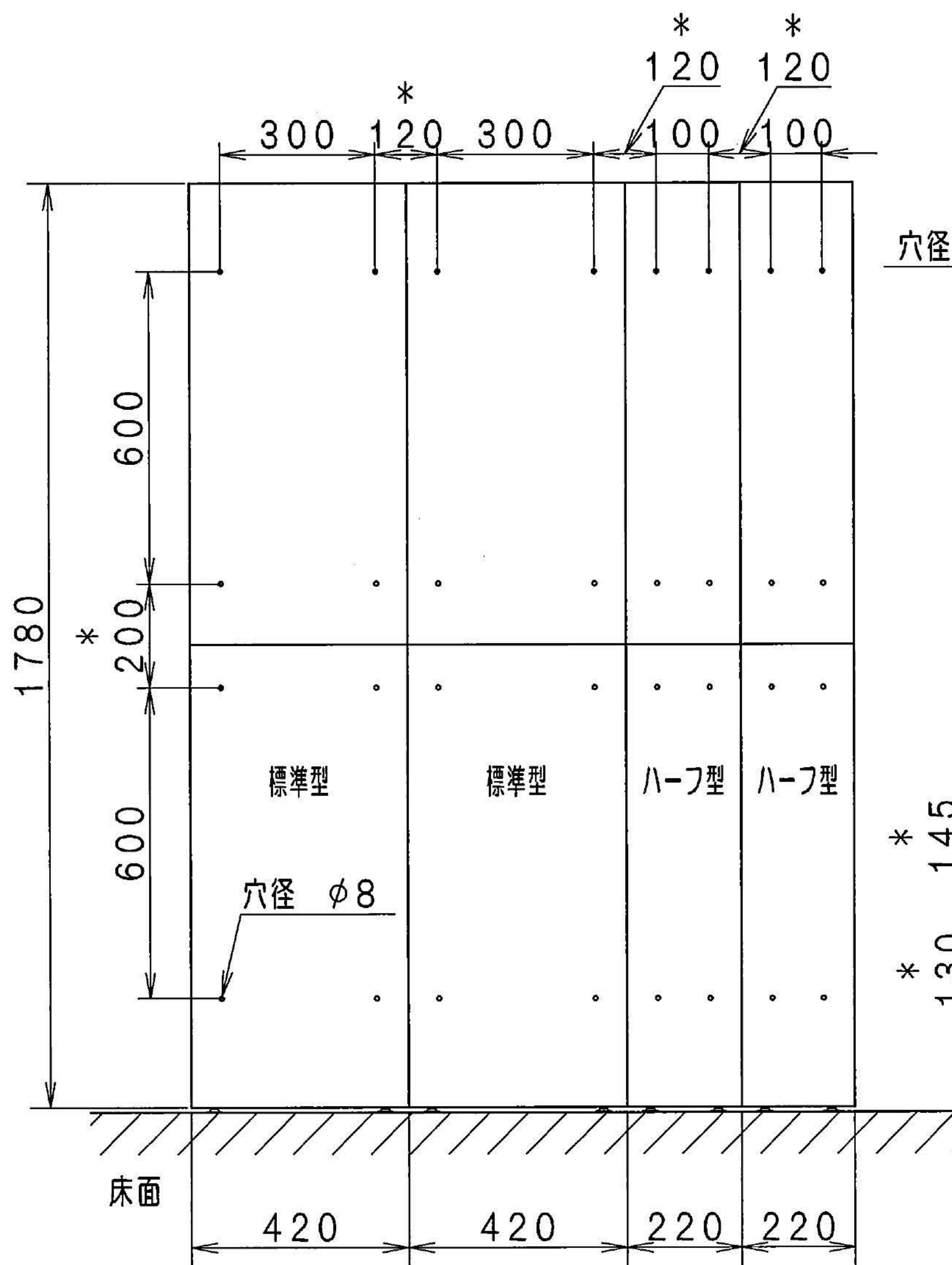
壁面アンカーピッチ図
