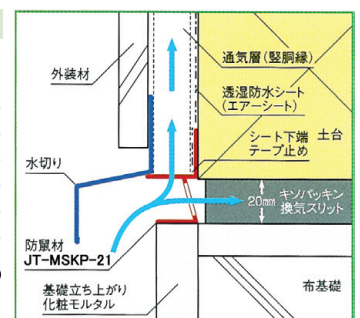
JT-MSKP-21の納まり図
