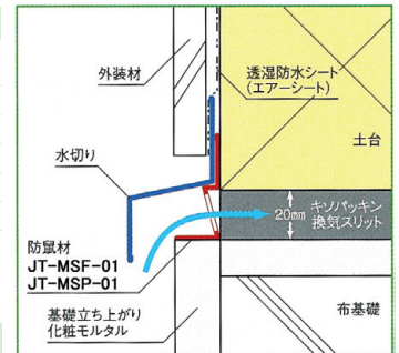
JT-MSF-01・JT-MSP-01の納まり図
