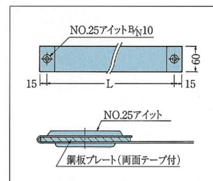
[FTB-A型] ガラスクロス+ アルミラミネート製 (防災1級合格品) 引張強度: 500kg/15mm
