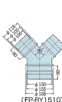
(FP-RY1510)
