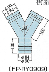
(FP-RY0909)
