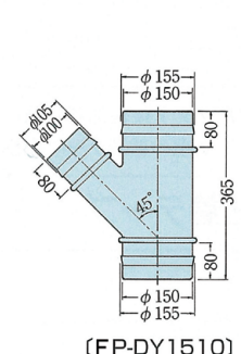
(FP-DY1510)
