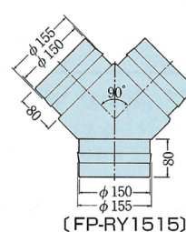
(FP-RY1515)
