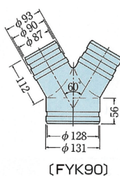
(FYK90)
