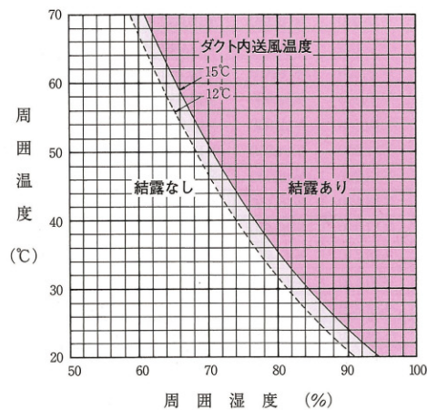
保温・防露効果(露点温度曲線)
