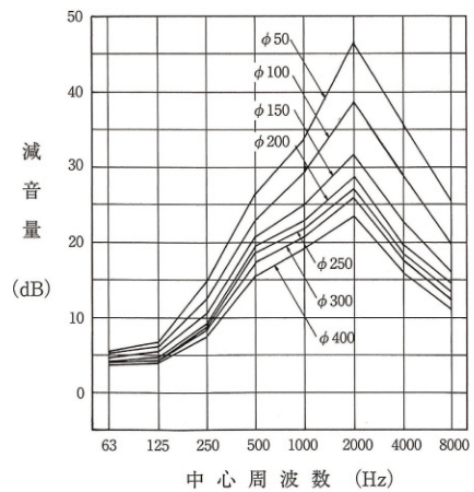
消音効果(1m)
