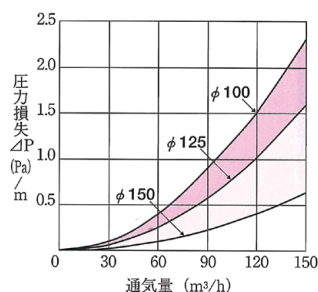
抵抗損失曲線
