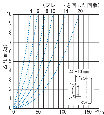
IM-10-OPK-K 通気量グラフ
