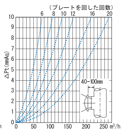
IM-15-OPK-K 通気量グラフ
