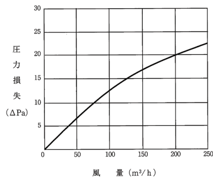
FTDD150抵抗曲線
