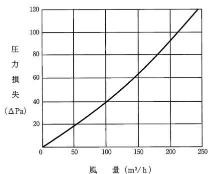
FTDD100抵抗曲線
