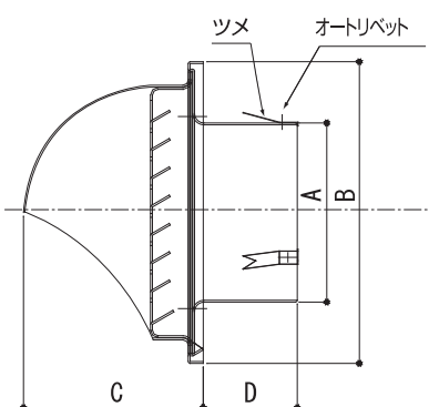
[縦断面図]
