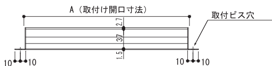
【外観図】
