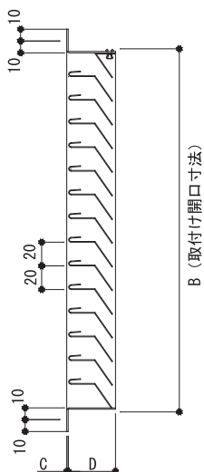
【縦断面図】
