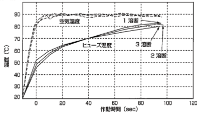
軒裏換気口LN-90・FD温度ヒューズ試験 試験番号55355号 作動試験
