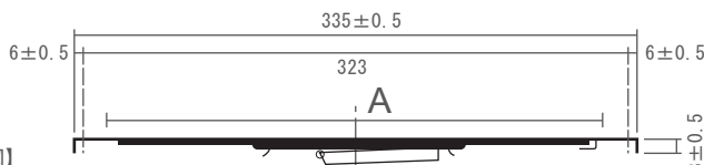
【断面図】
