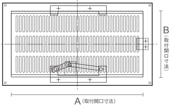
【裏面図】
