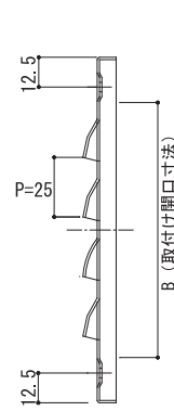
【縦断面図】
