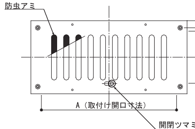
【外観図】
