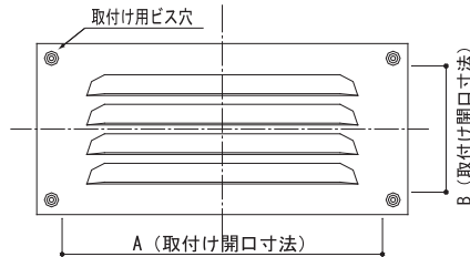
【外観図】
