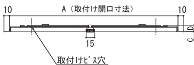
【外観図】
