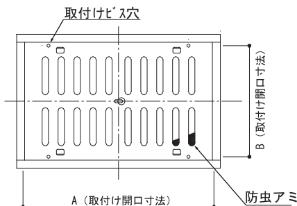
【外観図】
