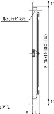
【縦断面図】
