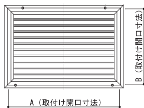
【外観図】
