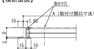
【横断面図】
