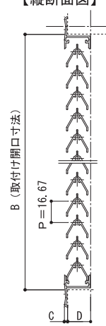
【縦断面図】
