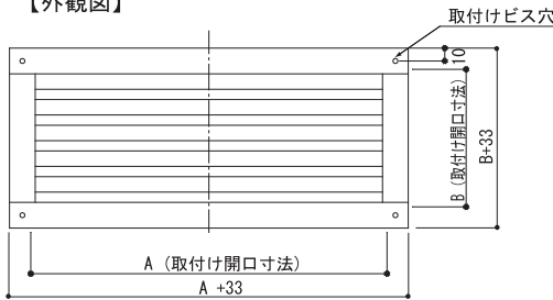
【外観図】
