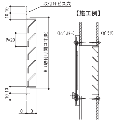
【縦断面図】
