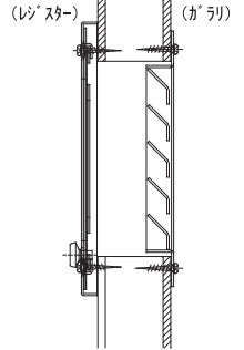
【施工例】
