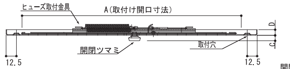
【外観図】
