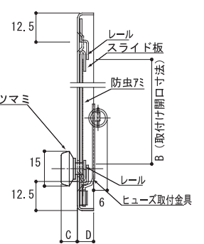
【縦断面図】
