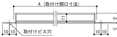
【外観図】
