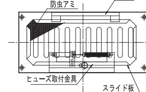
【内観図】
