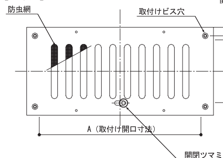
【外観図】
