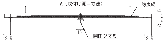
【外観図】
