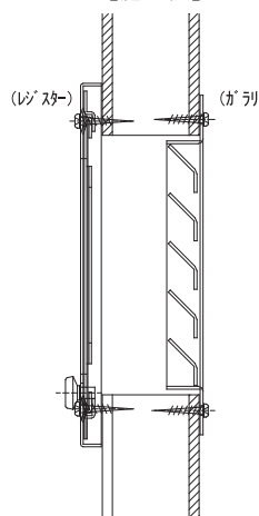
【施工例】
