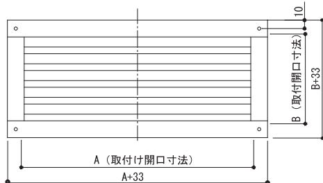
【外観図】
