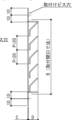
【縦断面図】
