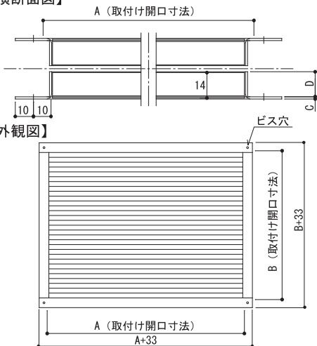
【横断面図】
