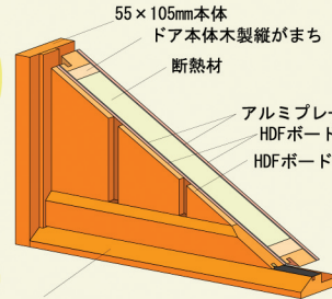
アルミ板付ハードウッド材敷居
